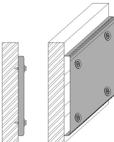
Rammschutz Typ 2+4
